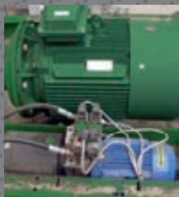
Centralina idraulica per gestione apertura portello dal PC
